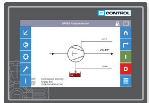
Дисплей B-CONTROL III
